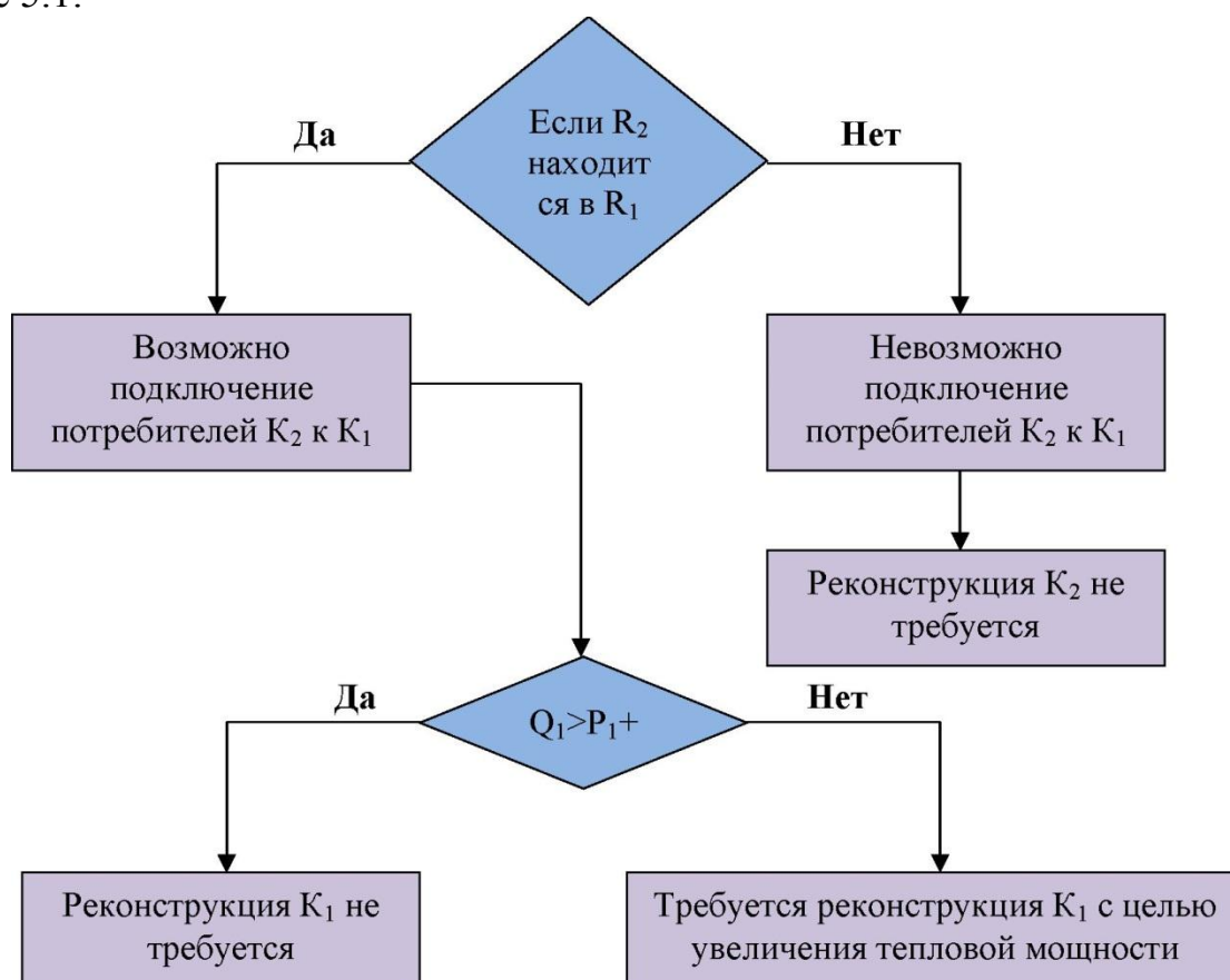
Рисунок 5.1 - Блок-схема обоснования реконструкции котельной K 2 , K 1 - котельная №1 и котельная №2;
